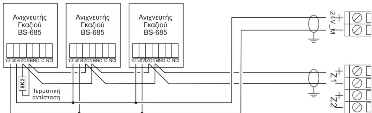
Σχήμα 4-7. Σύνδεση 3 ανιχνευτών αερίων BS-685 ή BS-686. Εκτός της σύνδεσης με τις κλέμες της ζώνης οι ανιχνευτές αυτοί πρέπει να τροφοδοτηθούν και με τάση από τις κλέμες 24V_M.
