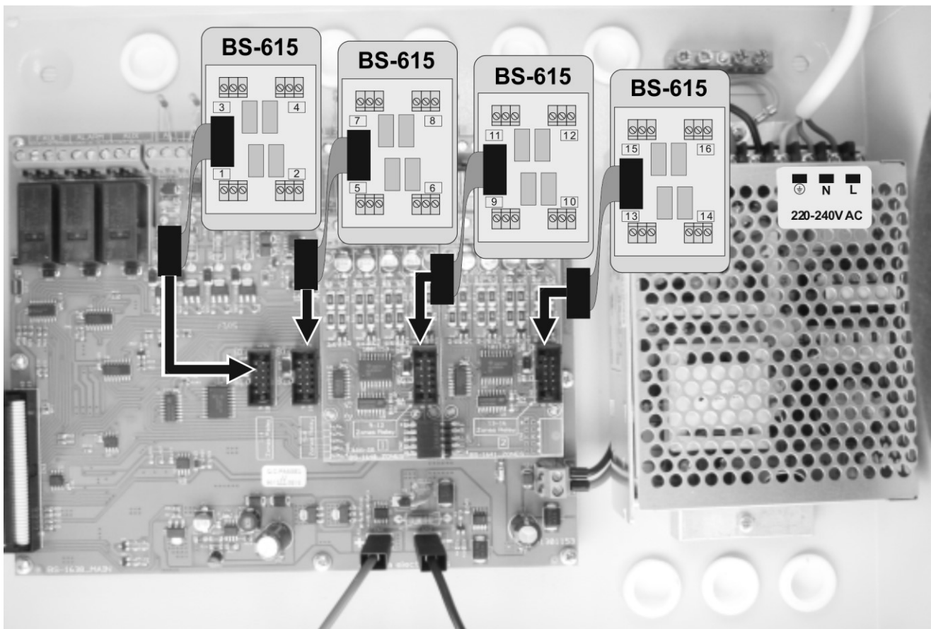
Σχήμα 4-9. Σύνδεση συσκευών BS-615.
