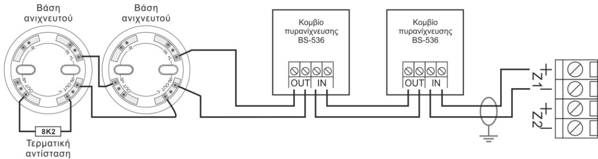
Σχήμα 4-6. Σύνδεση 2 βάσεων ανιχνευτών στη ζώνη 1 και 2 μπουτόν πυρανίχνευσης. Στην κάθε βάση μπορεί να τοποθετηθεί ανιχνευτής BS-655, BS-660 ή BS-657.
