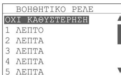
Σχήμα 5-6. Καθυστέρηση βοηθητικού ρελέ
