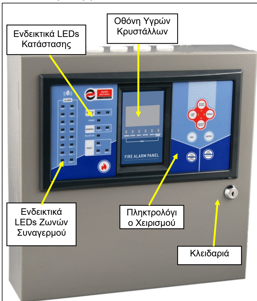
Σχήμα 1-1. Πρόσοψη πίνακα
