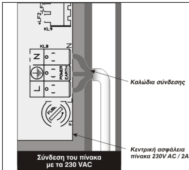
Σχήμα 3-5. Σύνδεση 230VAC
