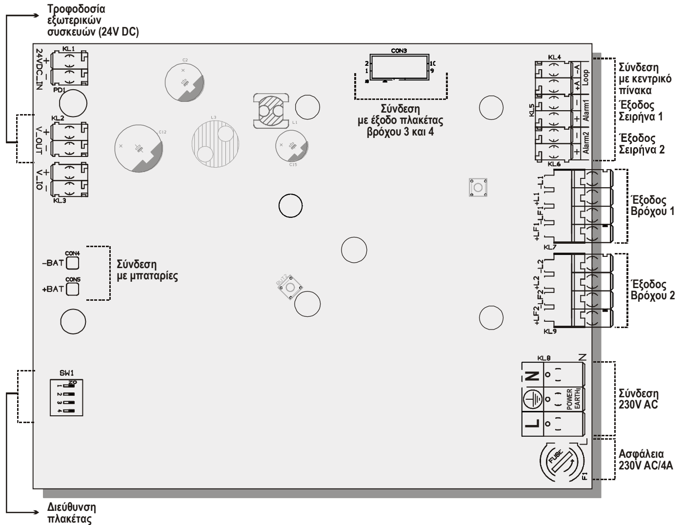
Σχήμα 3-2. Πλακέτα βρόχου
