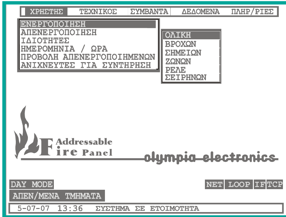
Σχήμα 4-7. Μενού Ενεργοποίηση
