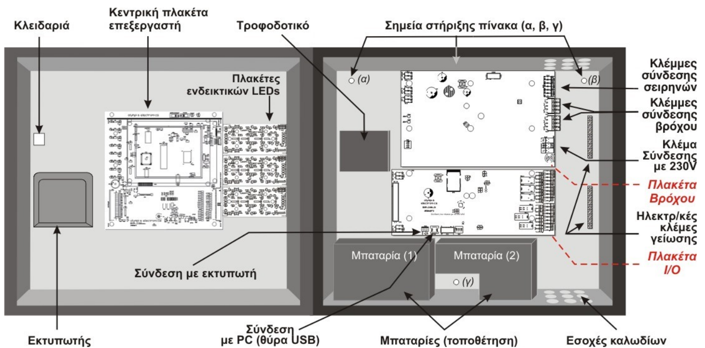
Σχήμα 3-1. Εσωτερικό πίνακα
