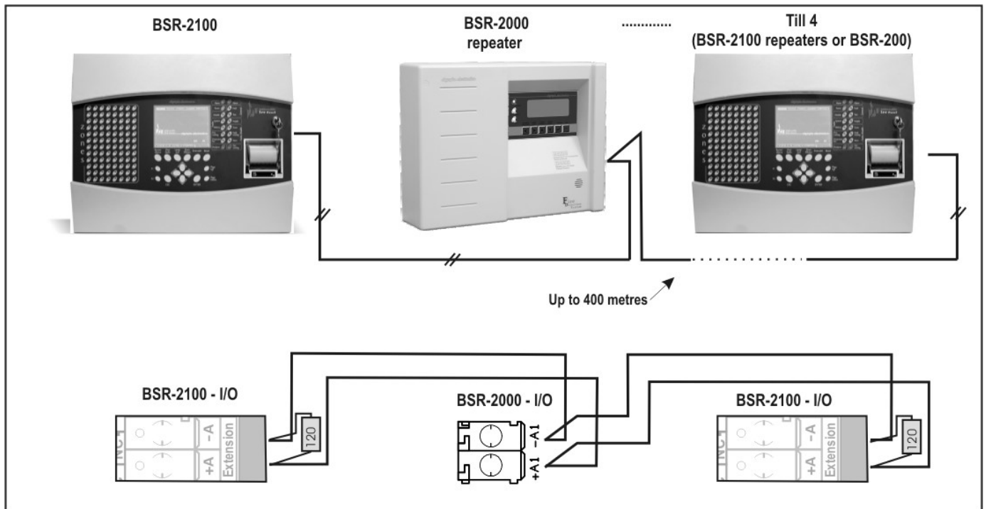
Σχήμα 3-14. Σύνδεση επαναλήπτη.
