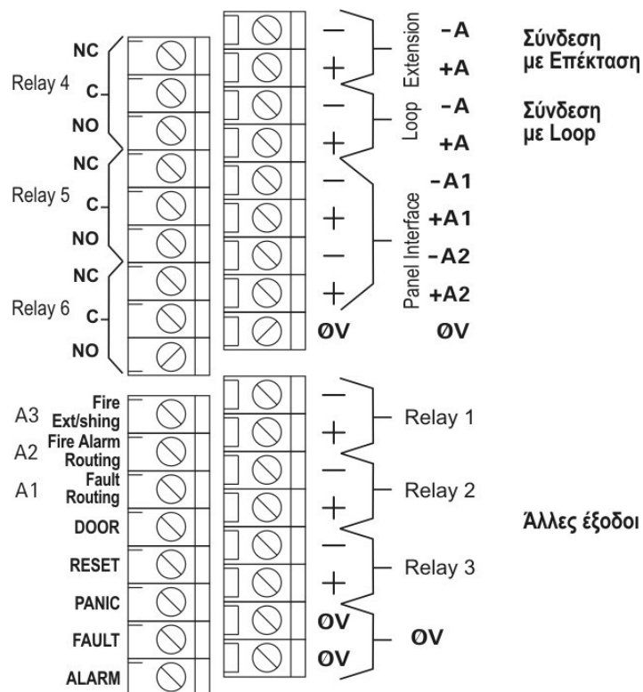
Σχήμα 3-3. Πλακέτα Εισόδου / Εξόδου
