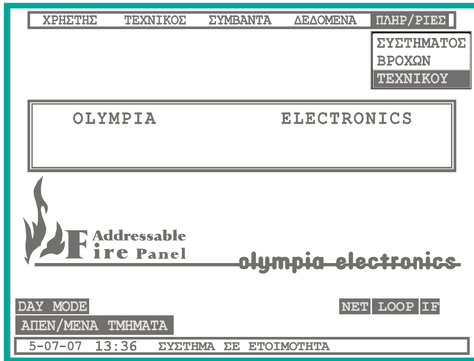
Σχήμα 4-32. Πληροφορίες τεχνικού
