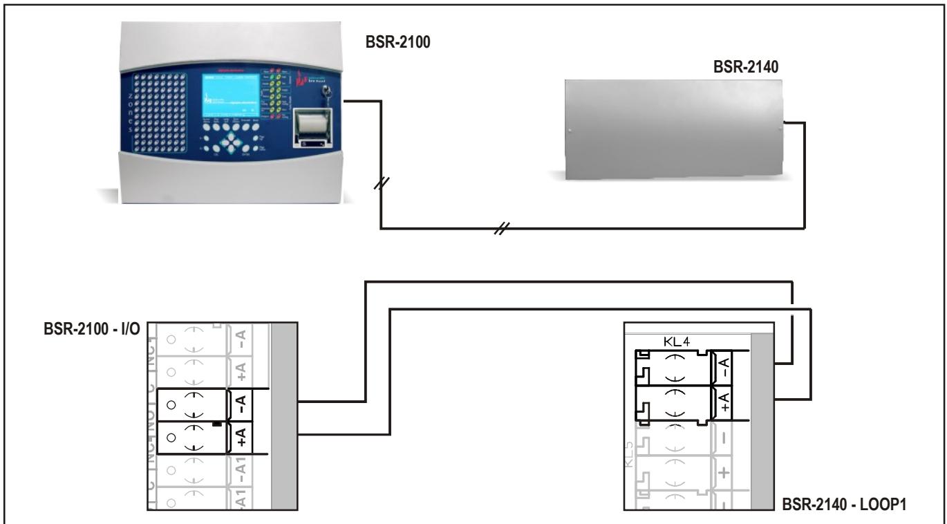
Σχήμα 3-13. Επέκταση βρόχων.
