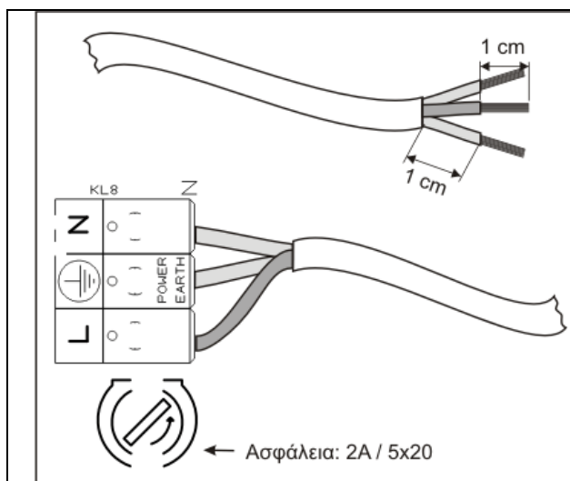
Σχήμα 3-6. Κλέμμη τροφοδοσίας 230VAC
