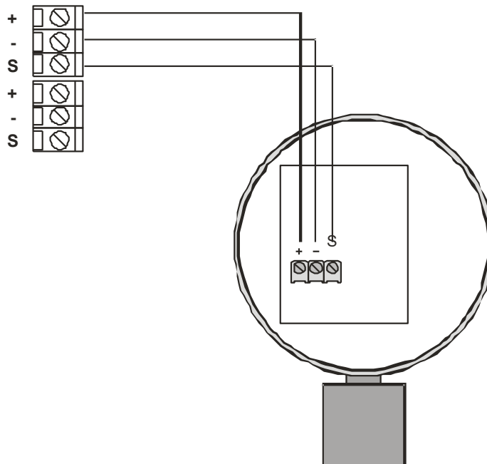
Σχήμα 4: Διάγραμμα σύνδεσης ανιχνευτών με τρεις επαφές
