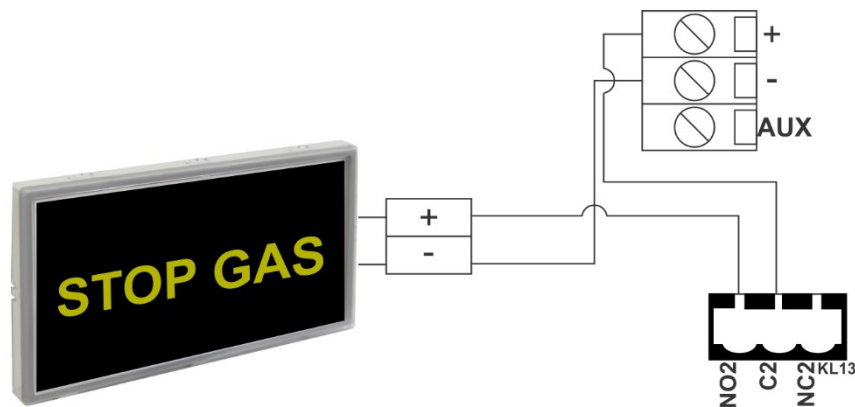
Σχήμα 6: Ενδεικτική σύνδεση φωτεινής ένδειξης με ρελέ του πίνακα.
