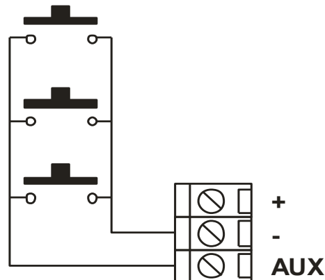
Σχήμα 5: Ενδεικτική σύνδεση ενεργοποίησης εισόδου.
