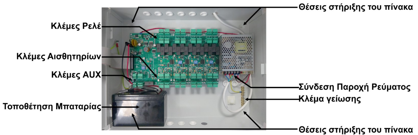
Σχήμα 2: Εσωτερικό του πίνακα
