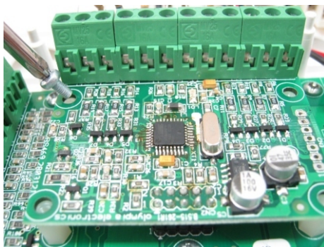
Σχήμα 5 : Βιδώμα της πλακέτας BS-469
