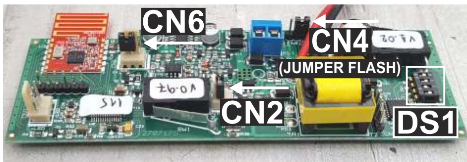
Φωτογραφία 4. Κεντρική πλακέτα σειρήνας.
