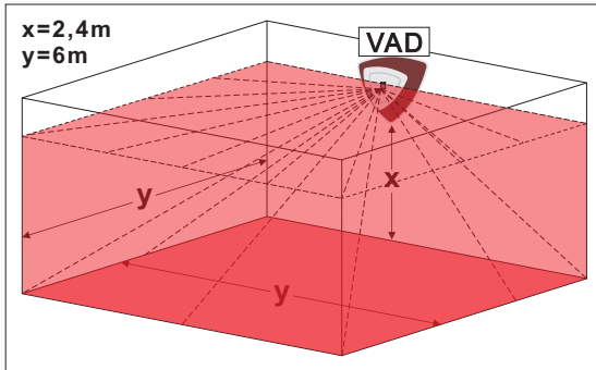
Σχήμα 1. Επιτοίχια Τοποθέτηση
