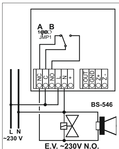
Σχεδιάγραμμα με χειροκίνητη επαναποθετούμενη κανονικά ανοιχτή ηλεκτροβάνα και φαρσοσειρήνα 230VAC
