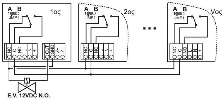
Σχήμα 3B.Σύνδεση ανιχνευτών αερίου σε δίκτυο με μια ηλεκτροβάνα 12VDC N.O.
