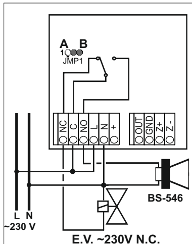
Σχεδιάγραμμα με χειροκίνητη επαναποθετούμενη κανονικά κλειστή ηλεκτροβάνα και φαρσοσειρήνα 230VAC
