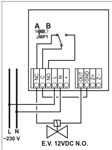
Σχεδιάγραμμα με χειροκίνητη επαναποθέτηση και κανονικά ανοιχτή ηλεκτροβάνα
