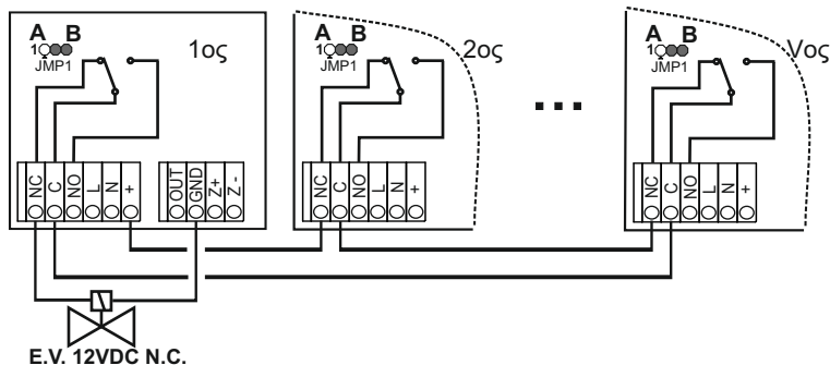
Σχήμα 3Α. Σύνδεση ανιχνευτών αερίου σε δίκτυο με μια ηλεκτροβάνα 12VDC N.C.
