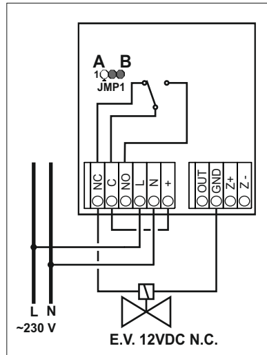
Σχεδιάγραμμα με χειροκίνητη επαναποθέτουμένη και κανονικά κλειστή ηλεκτροβάνα
