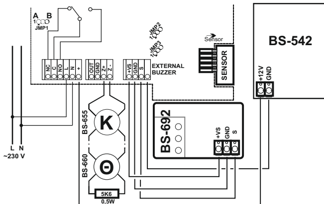
Σχήμα 2. Σχεδιάγραμμα σύνδεσης εξωτερικών συσκευών
