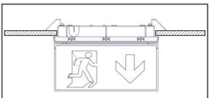
Χωνευτή τοποθέτηση με εξαρτήματα στήριξης και πινακίδα σήμανσης
