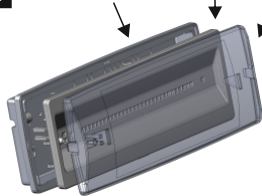
1 Kunststoffbasis Reflektor Diffusor
